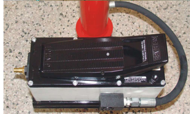
pneumaticko-hydraulický agregát
